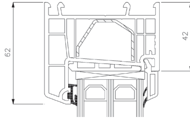
Oberrahmen
