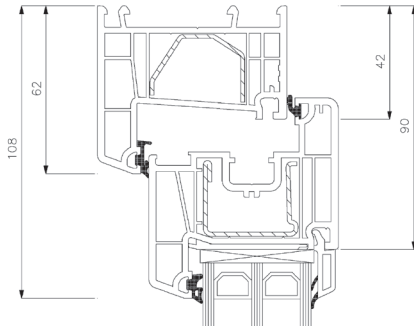
Oberrahmen
