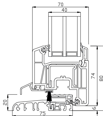
Bodenschwelle Aluminium
