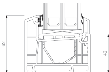
Unterrahmen
