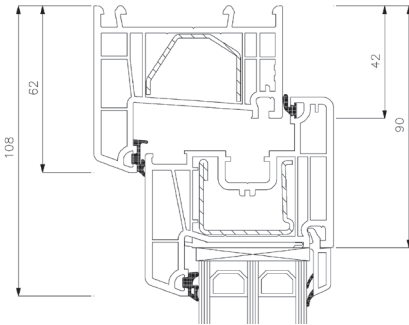
Seitenrahmen
