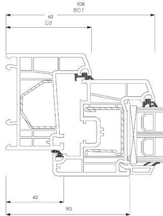
Seitenrahmen
