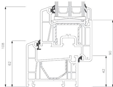
PVC Unterrahmen
