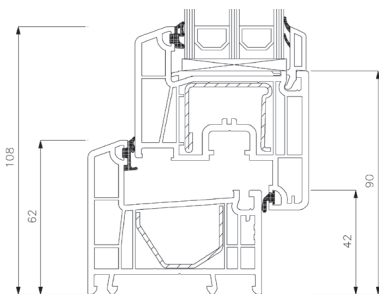
Unterrahmen
