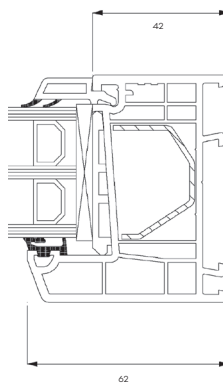
Seitenrahmen
