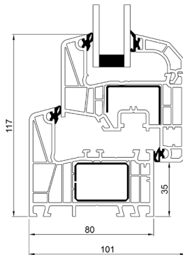
PVC Unterrahmen
