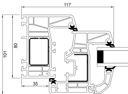
Unterrahmen
