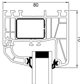
Oberrahmen
