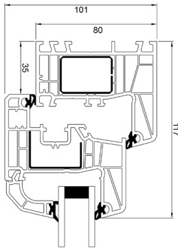
Seitenrahmen
