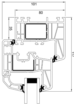
Oberrahmen
