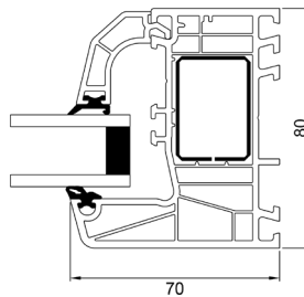
Seitenrahmen
