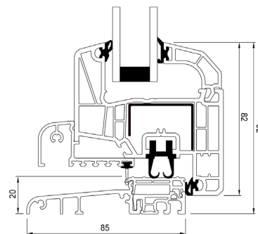
Bodenschwelle Aluminium
