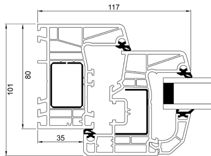
Seitenrahmen
