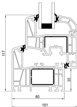
Unterrahmen
