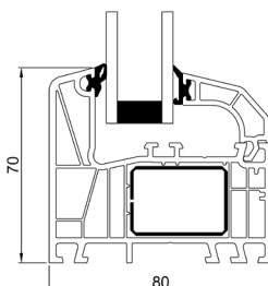
Unterrahmen
