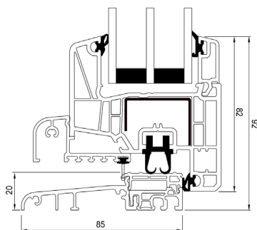
Bodenschwelle Aluminium
