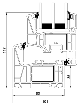
PVC Unterrahmen
