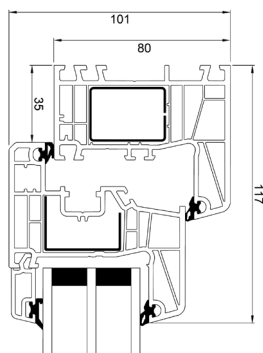
Oberrahmen
