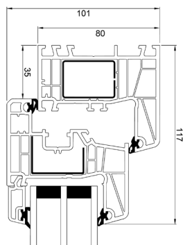
Seitenrahmen
