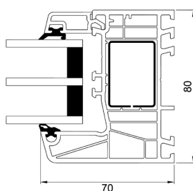
Seitenrahmen
